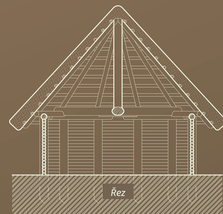
Konstrukce střechy
