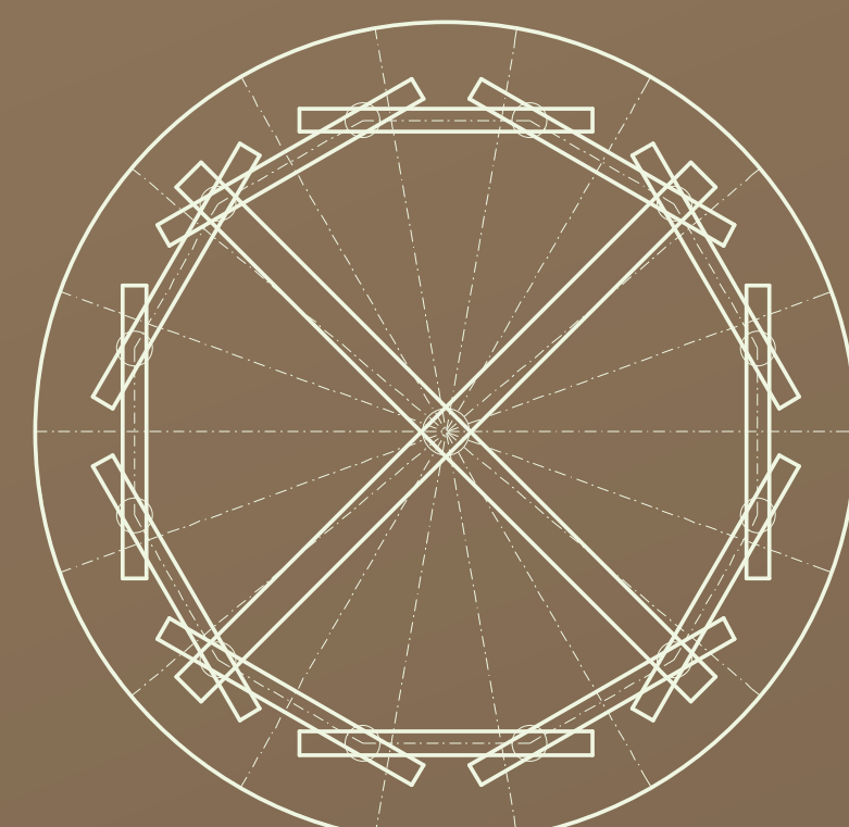
Konstrukce střechy
